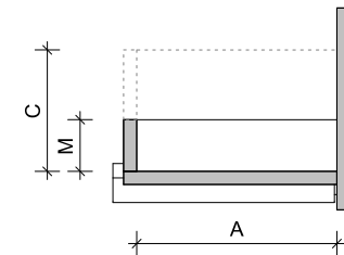
Schubkasten (Auszug)
