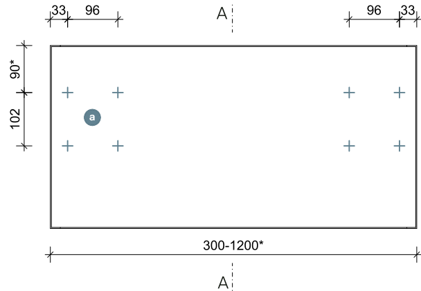
DRAUFSICHT
