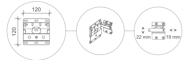
Hängende Befestigung mit Wandmontageplatte und Schwerlastaufhängern
