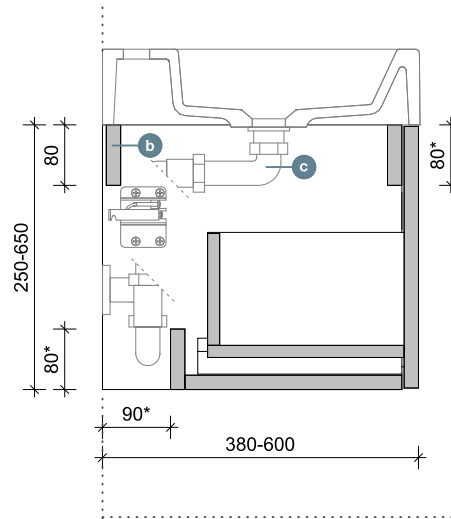
SNITT A-A (Beispiel mit Waschbecken und Raumsparnsiphon)
